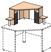
28P700 применяется со столом 28S700 842x842x472
